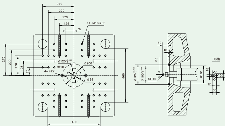
• UN160A2
