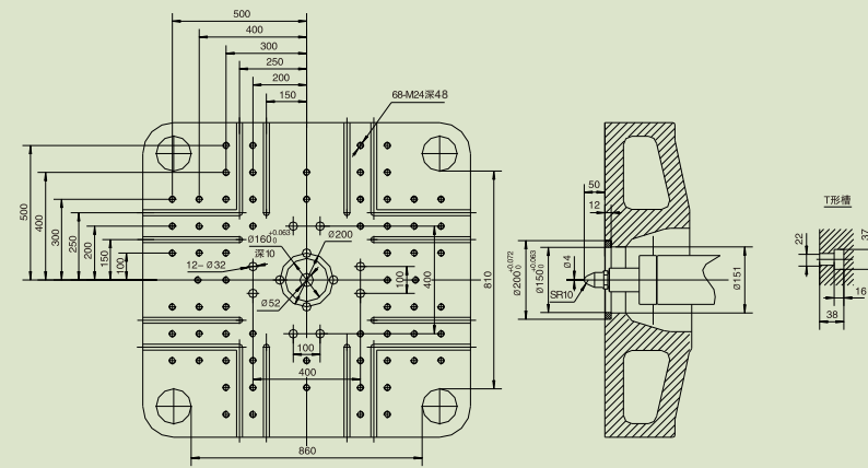
• UN480A2
