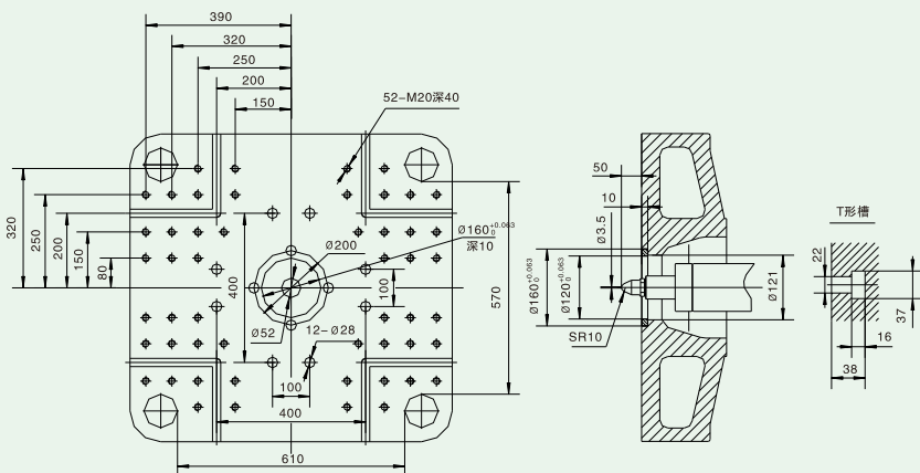
• UN260A2
