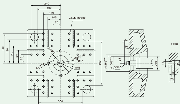
• UN90A2
